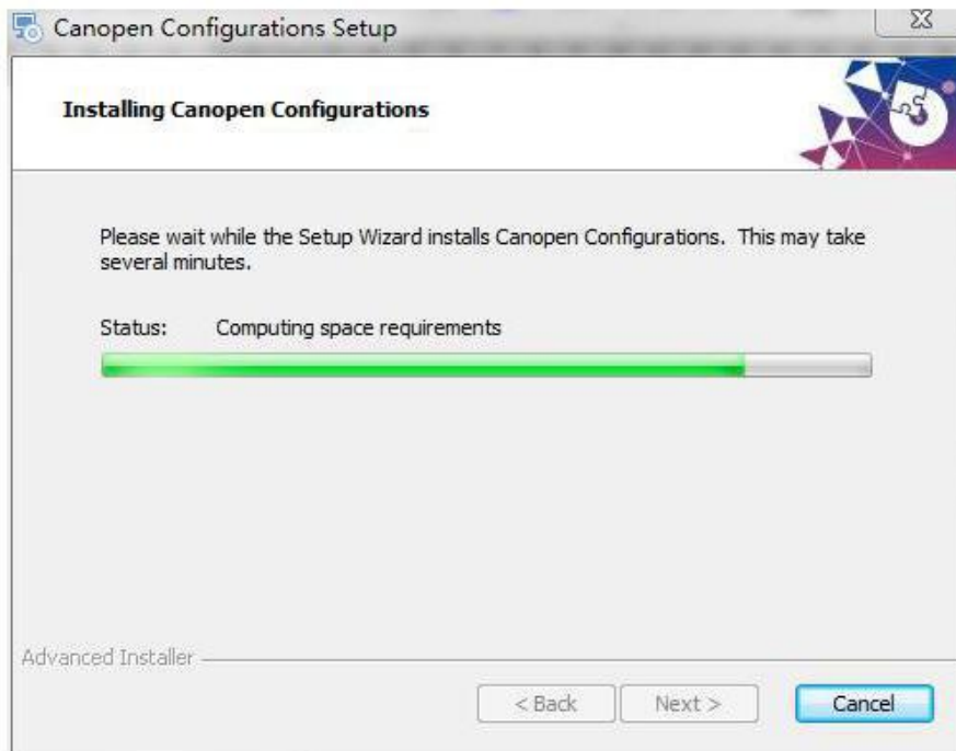
图 4.17 正在安装
