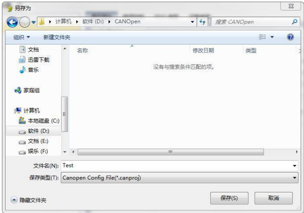
图 4.35 保存配置
