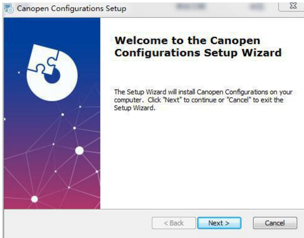
图 4.15 准备安装
