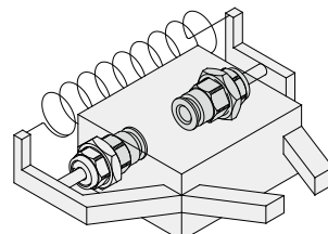
夾爪
