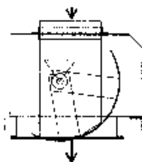
圆弧门给料
