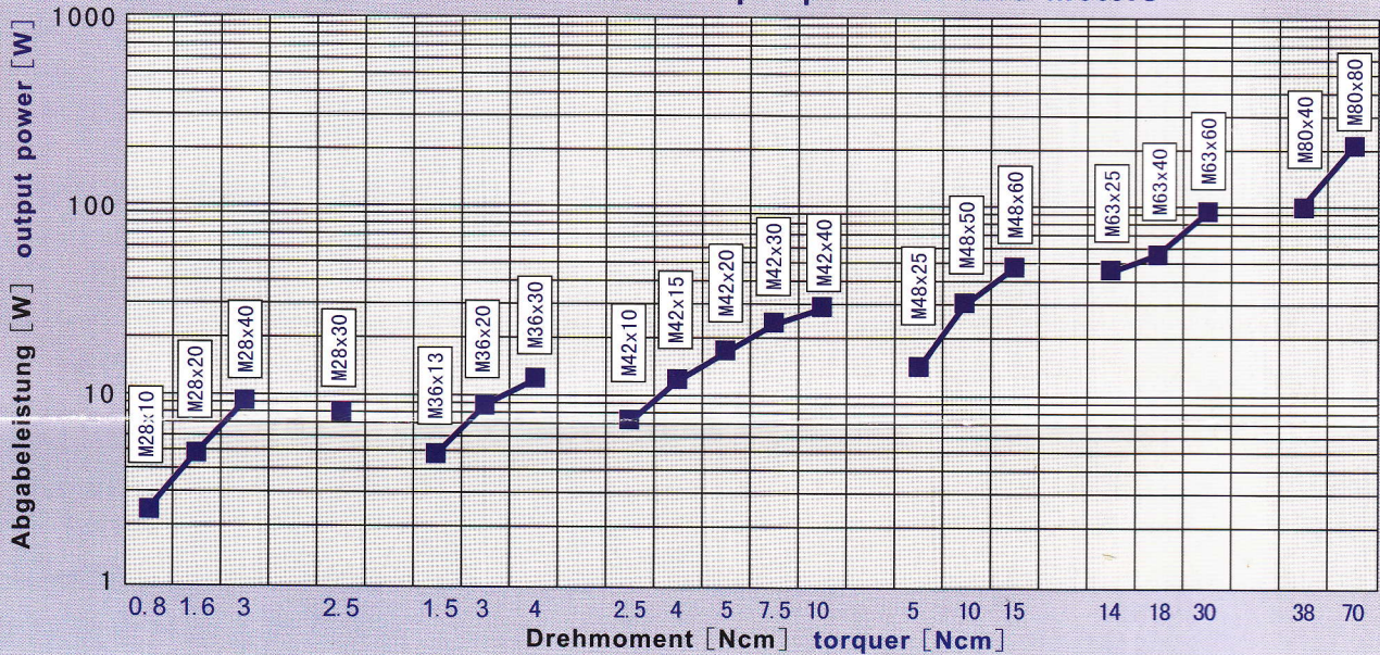
Zulässige Dauerabgabeleistung der KAG-Motoren Permissible continuous output power of KAG motors
